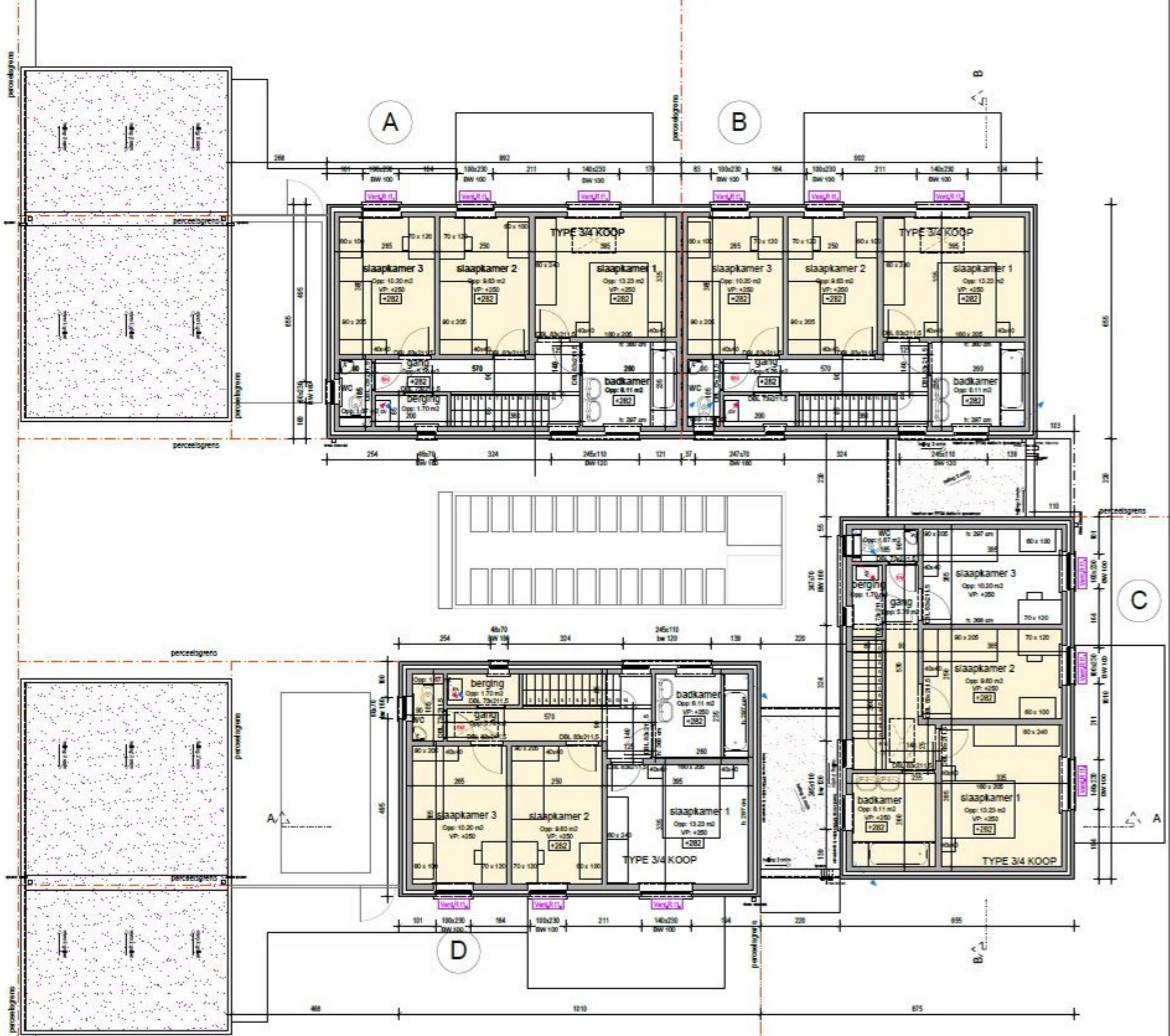
Grondplan verdieping schaal 1/50
