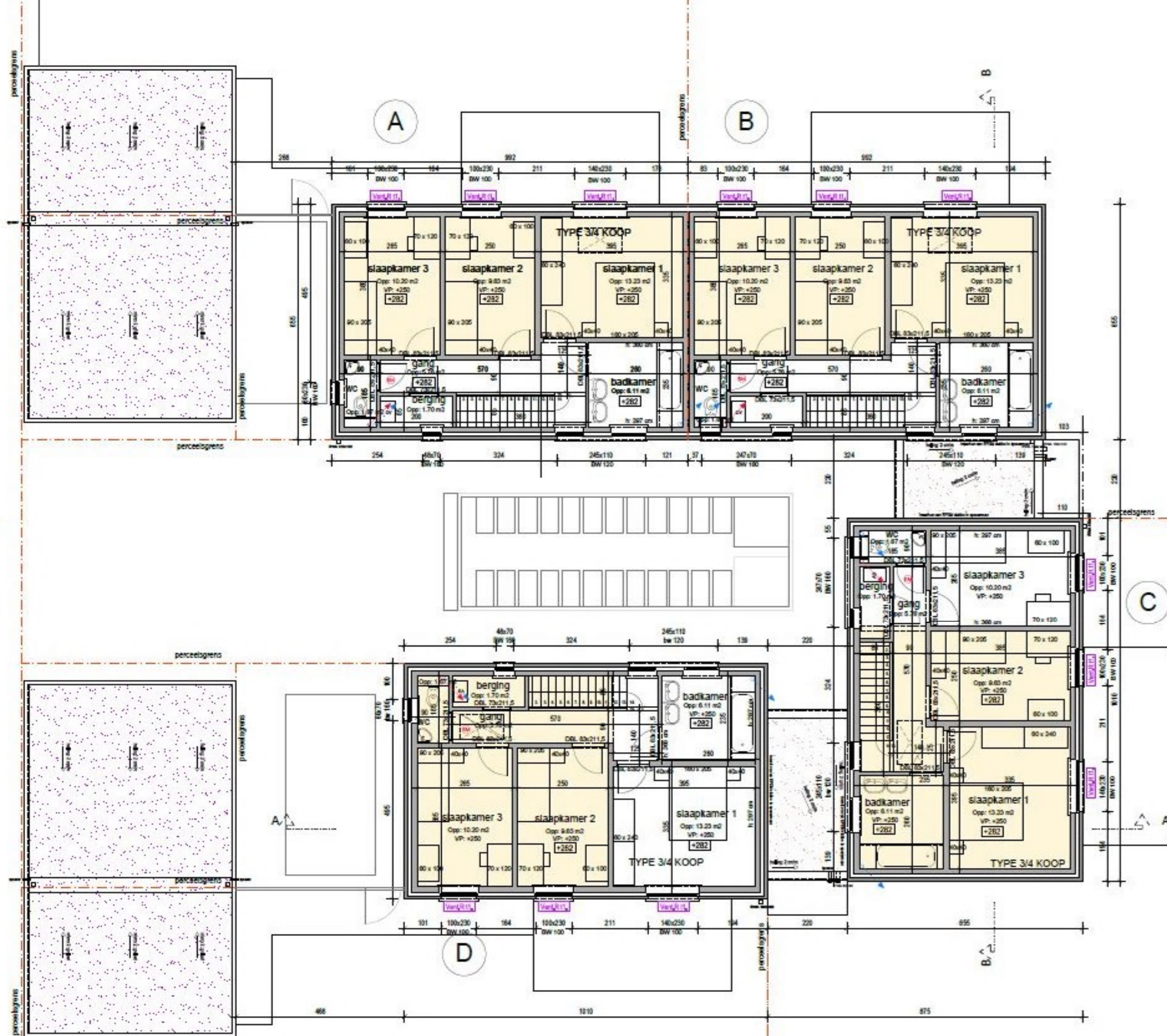
Grondplan verdieping schaal 1/50
