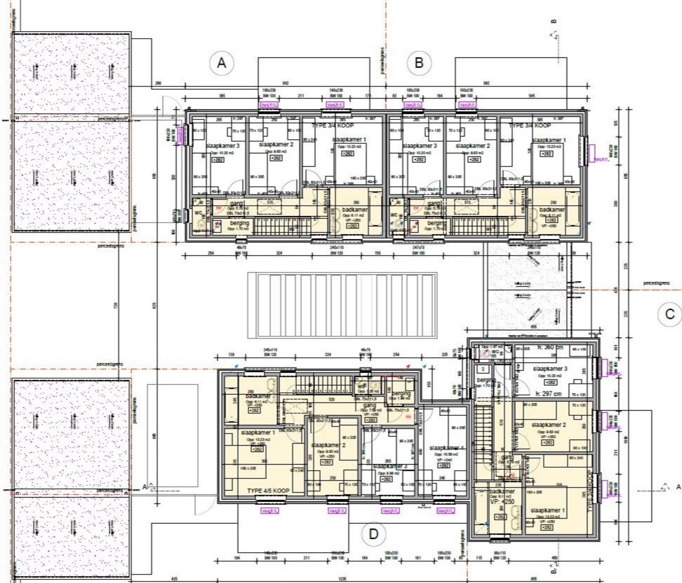
Grondplan verdieping schaal 1/50
