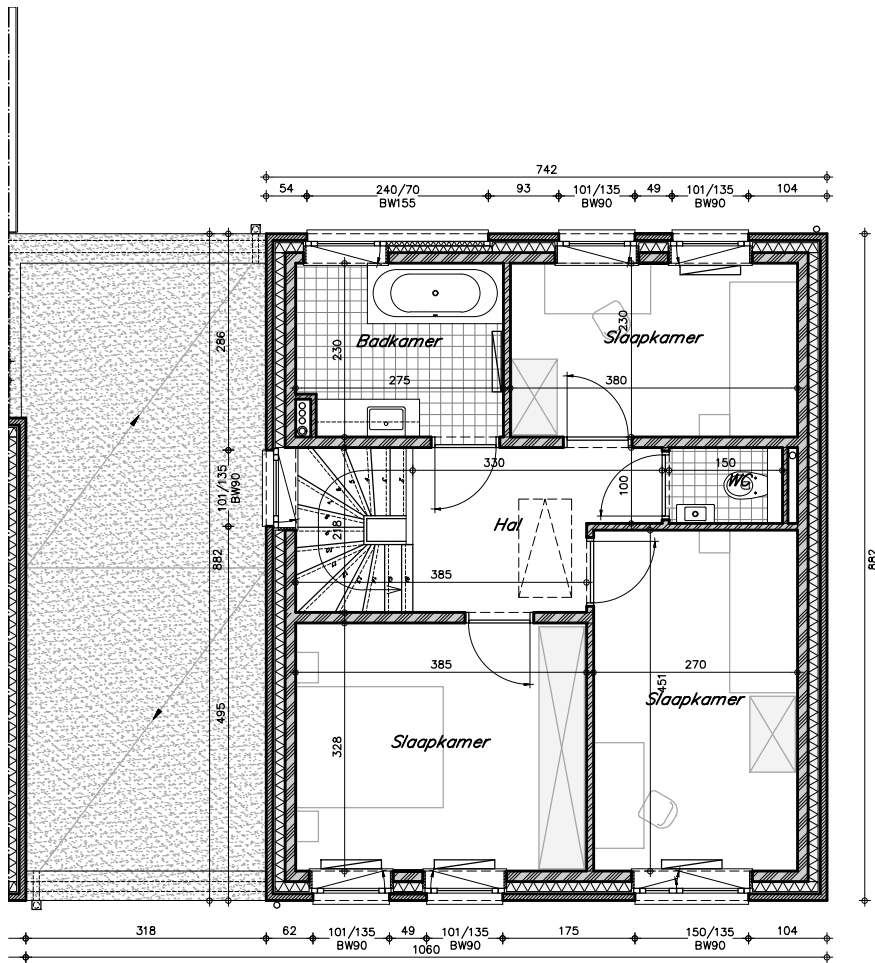
Verdiepingsplan
